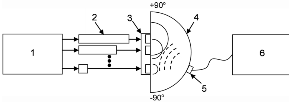
Рис. 2. Схема вимірювання ПЧХ лінійної ФАР ПЕП на основі методу з сумісним збудженням п'єзоперетворювачів в режимі випромінювання імпульсних сигналів:
