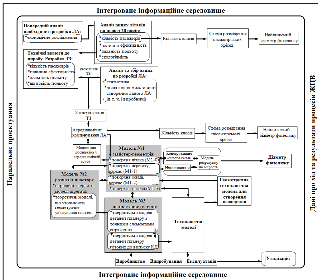
Рис. 2. Схема життєвого циклу ла та місце в ньому фюзеляжу літака: тз – технічне завдання; кд – конструкторська документація
