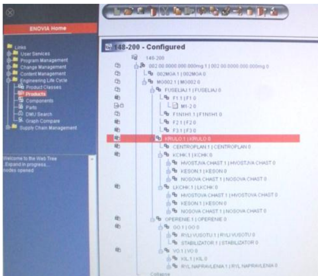
Рис.5. База даних складових життєвого циклу літального апарату
