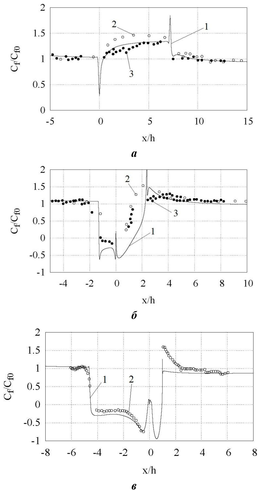
Рис. 3. Порівняння експериментальних та розрахункових значень C_f / C_{f0} : a – кут нахилу 8^\circ ; б – кут нахилу 25^\circ ; в – кут нахилу 90^\circ ; 1 – розрахункові значення; 2 – експериментальні значення для h=15 мм; 3 – експериментальні значення для h=6 мм
