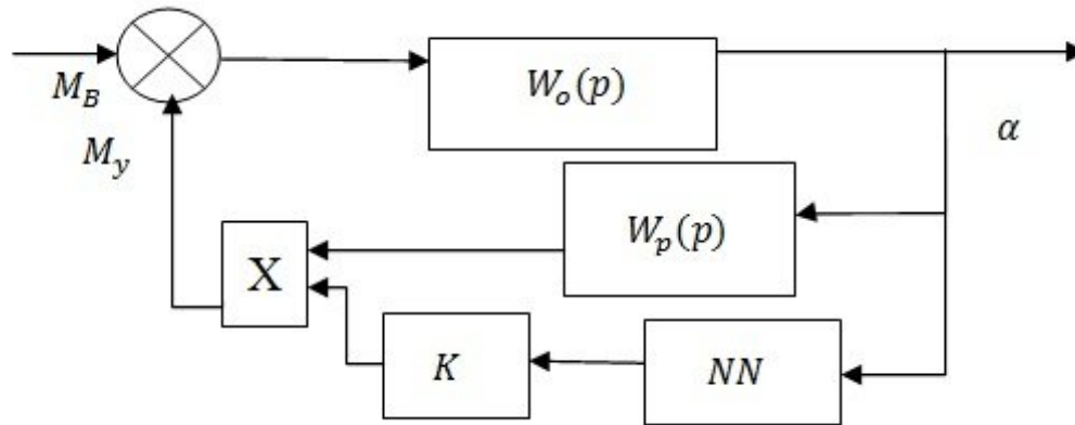
Рис. 1. Структурная схема адаптивной системы управления
