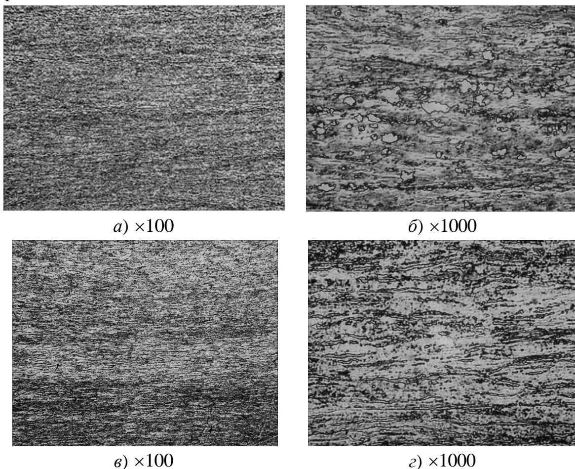
Рис. 1. Микроструктура горячепрессованных труб двух производителей ( a, б – производитель № 1; в, г – производитель № 2)
