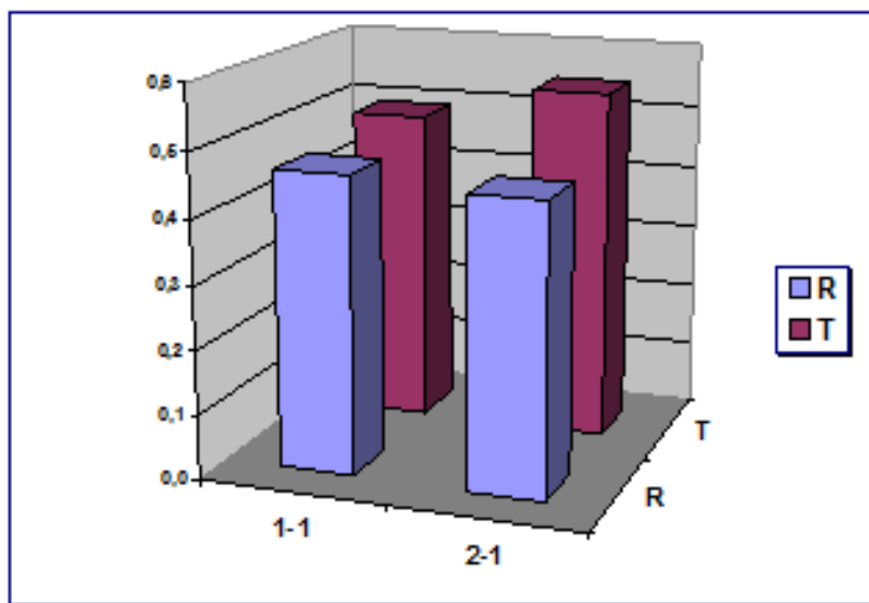
Рис. 2. Обратные полюсные фигуры (ОПФ) горячепрессованной заготовки 1-1, 2-1 (верхние рисунки) и диаграмма соответствующих значений текстурного параметра
